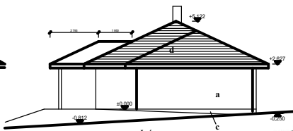
POHLED BOČNÍ - východní
