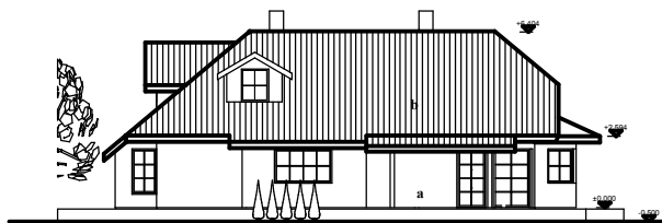
POHLED BOČNÍ - západní
