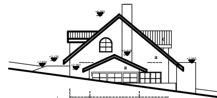
POHLED BOČNÍ - Západ
